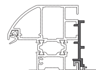
Profilé complémentaire de recouvrement du doublage
