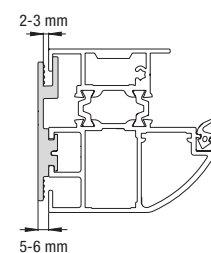
Huissérie en aluminium A1 avec bride de fixation pour Thermo46
