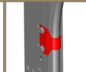
RACCORD D'ALIGNEMENT RAIL
