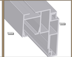
RAIL DE GUIDAGE MONOBLOC BLANC
