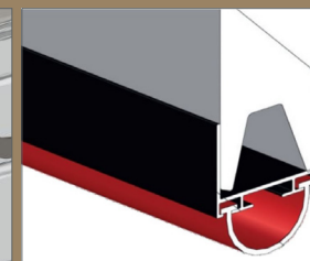
JOINT INFÉRIEUR CAOUTCHOUC
