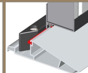
SEUIL BAS EN ALUMINIUM DRAINÉ
