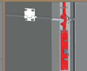
SERRURE À CROCHETS HAUTE ET BASSE
