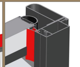
JOINT TUBULAIRE À LÈVRES CÔTÉ FERMETURE
