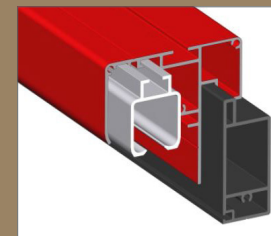
PRÉCADRE NOIR AVEC PROFIL DE RAIL MONOBLOC
