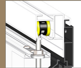
CHARIOT 4 ROULETTES SUR ROULEMENT AXE EN INOX
