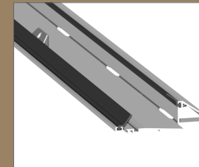
SEUIL DRAINANT AVEC RESERVOIR D'EAU
