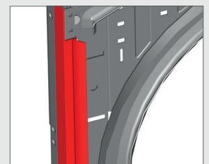
Joint à lèvres EPDM sur rails verticaux
