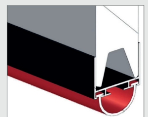
Joint à bulle EPDM sur panneau bas
