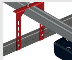
Assemblage et système easyfixe
