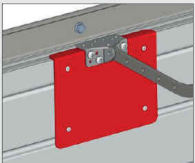
Plaque renfort pour liaison du bras moteur
