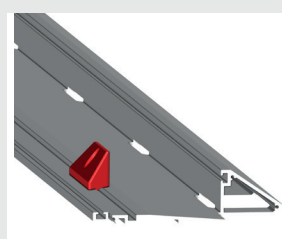
Patin de guidage en polyamide permettant une compression parfaite
