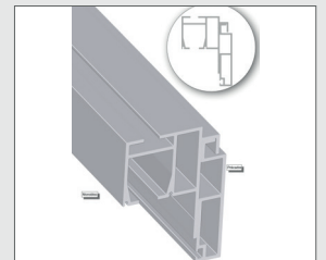
Rail de guidage supérieur blanc intégré dans le mono bloc
